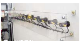
图 3 环氧挡板
